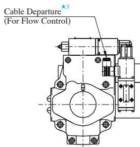
View Arrow Y
